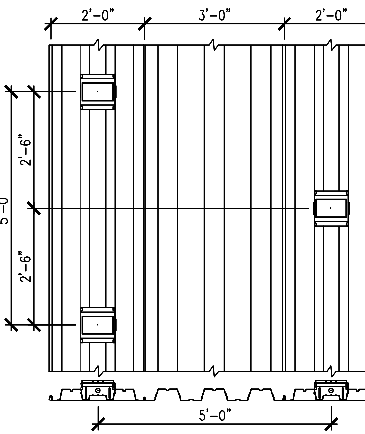
8 S1 N-R-G-FLO+ PRESET MODULE SCALE: 1" = 1'-0"
