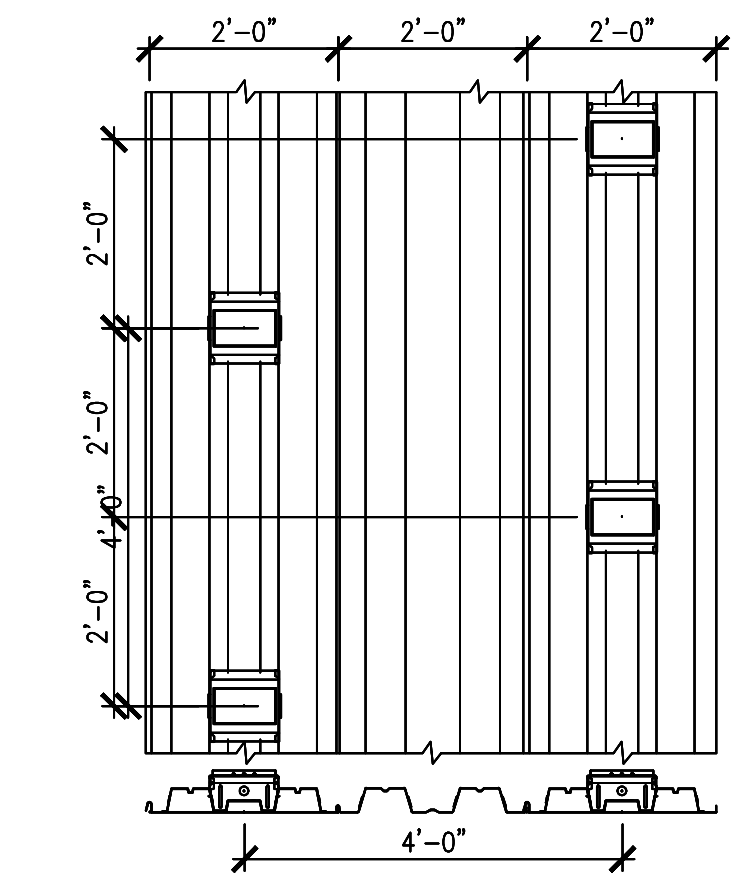
7 S1 N-R-G-FLO+ PRESET MODULE SCALE: 1" = 1'-0"
